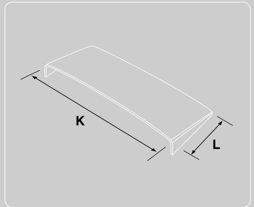
図3 (リアウイング寸法)
