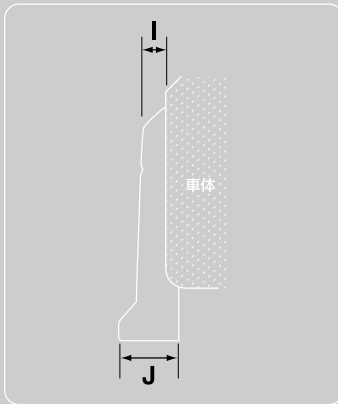
図2 (サイドステップ断面寸法)
